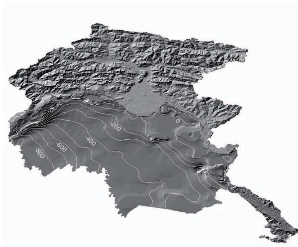
Ricostruzione del substrato pre quaternario della Pianura Friulana.
