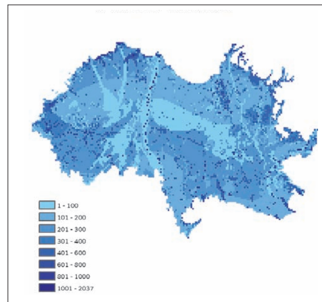
Distribuzione areale del valore della componente di ruscellamento superficiale (parametro R) espressa in mm/anno.
