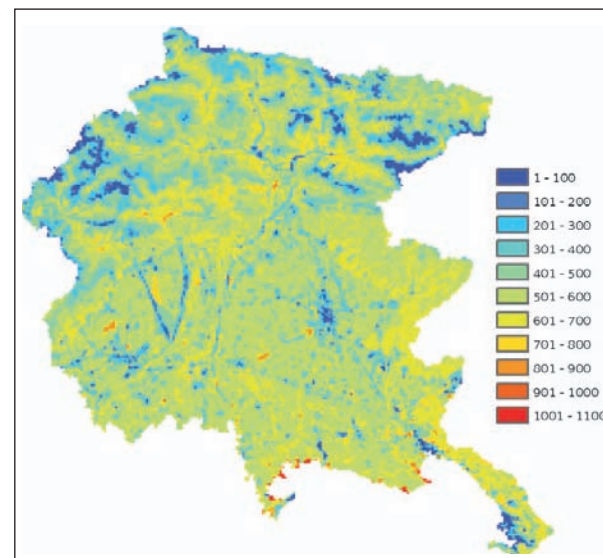
Distribuzione areale dei valori di evapotraspirazione colturale media annua (parametro Et) espressi in mm/anno.
