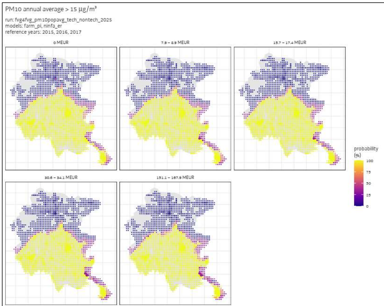
Figura 18: probabilità che nel 2025 non sia rispettata la media annuale di 15 \mu\text{g}/\text{m}^3 di \text{PM}_{10} (in giallo le aree più critiche). Ogni pannello corrisponde a un budget diverso, investito nella riduzione delle emissioni.
