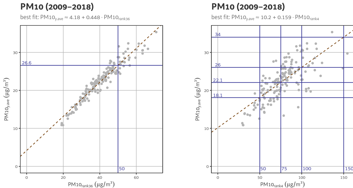
Figura 3: Relazione tra media annua e 36° (a sinistra) o 4° (a destra) valore giornaliero massimo per le stazioni FVG nel periodo 2009–2018. Ogni pallino grigio rappresenta il dato annuo di una stazione; la linea tratteggiata è il fit lineare descritto dalle equazioni riportate sopra ciascun grafico; le linee blu verticali individuano la soglia di legge sul 36° valore massimo (nel pannello a sinistra) o i livelli che l'OMS raccomanda di non superare più di tre giorni in un anno (nel pannello a destra); le linee blu orizzontali rappresentano le soglie equivalenti approssimative per la media annua.
