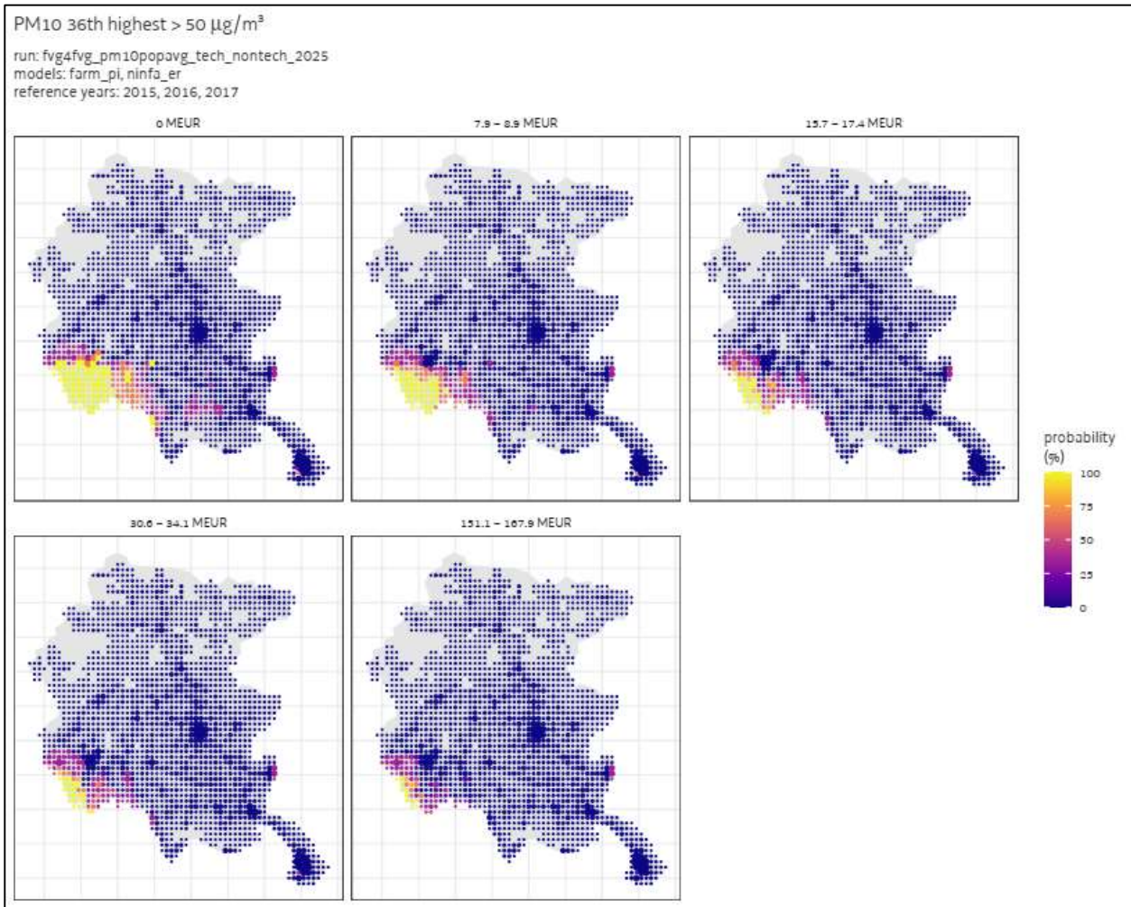
Figura 14: probabilità che nel 2025 non sia rispettato il limite dei 35 superamenti giornalieri di 50 µg/m 3 di PM 10 (in giallo le aree più critiche). Ogni pannello corrisponde a un budget diverso, investito nella riduzione delle emissioni.
