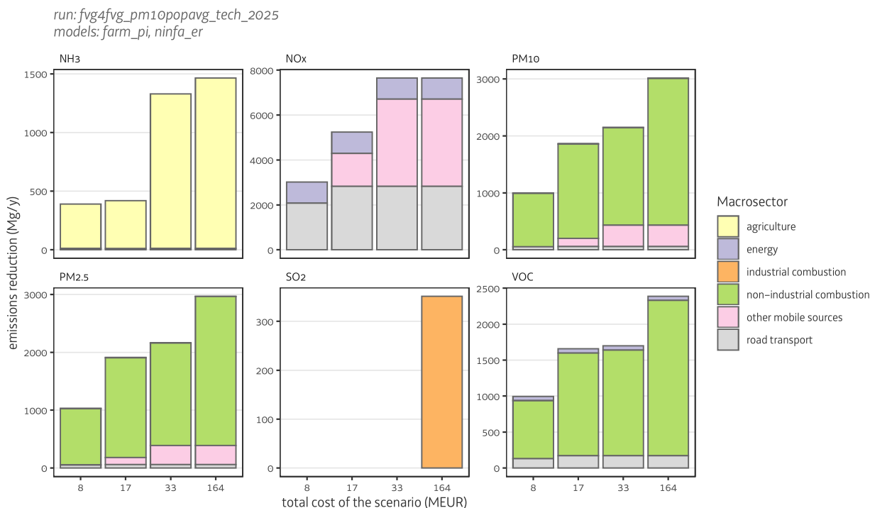
Figura 11: Riduzioni emissive ottenute con la strategia fvg4fvg_tech.
