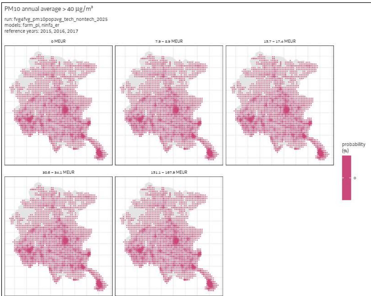
Figura 15: probabilità che nel 2025 non sia rispettata la media annuale di 40 µg/m 3 di PM 10 (non risultano aree critiche). Ogni pannello corrisponde a un budget diverso, investito nella riduzione delle emissioni.
