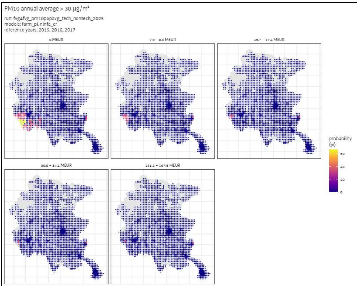
Figura 16: probabilità che nel 2025 non sia rispettata la media annuale di 30 µg/m 3 di PM 10 (in giallo le aree più critiche). Ogni pannello corrisponde a un budget diverso, investito nella riduzione delle emissioni.
