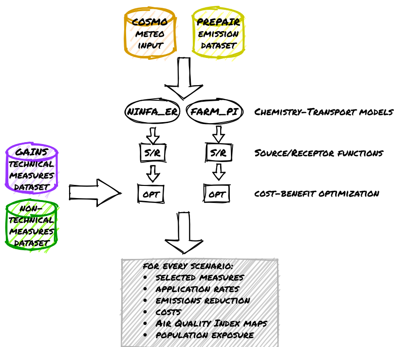
Figura 1: Schema di funzionamento di RIAT+ nella sua applicazione al nord Italia
