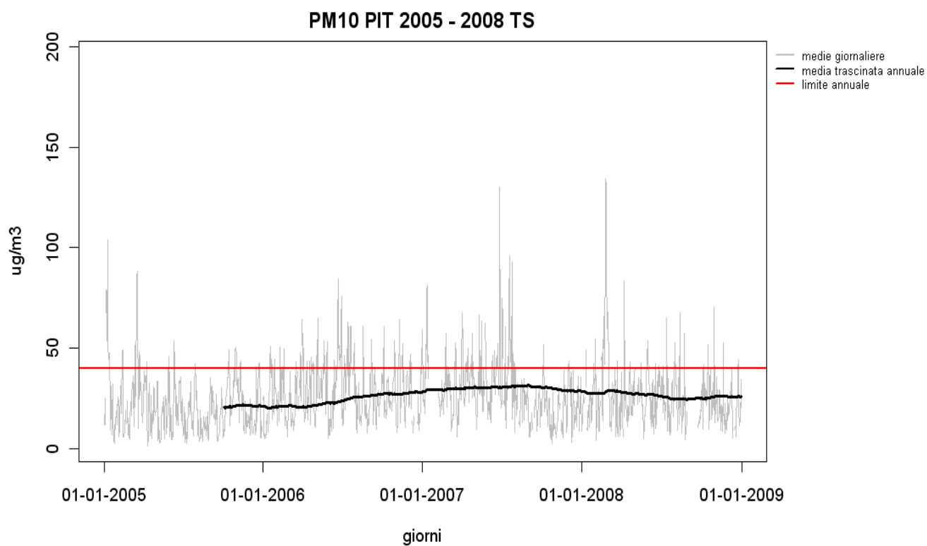
Figura 32 - Andamento delle medie trascinate annue nel periodo 2005-2008 nella stazione di via Pitacco.
