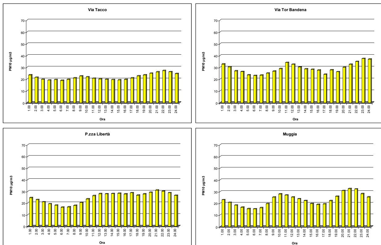
Figura 68: andamento medio orario (13/07/2007 – 11/11/2008) delle polveri sottili nelle stazioni più distanti rispetto alla ferriera di Servola.
