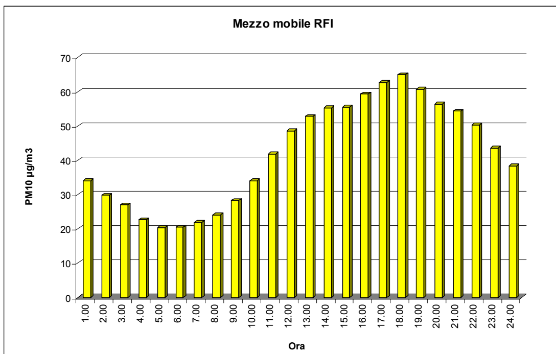
Figura 66: andamento medio orario (13/07/2007 – 11/11/2008) delle polveri sottili nella stazione RFI.
