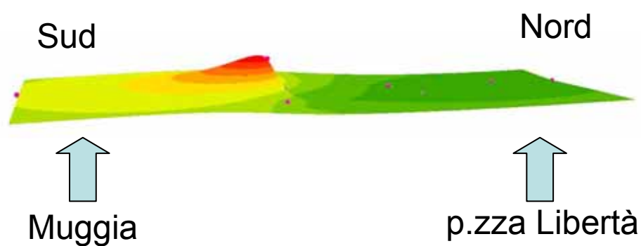
Figura 70:17/07/2007 - interpolazione dei valori di PM10 sull'area monitorata dalle centraline di ARPA
