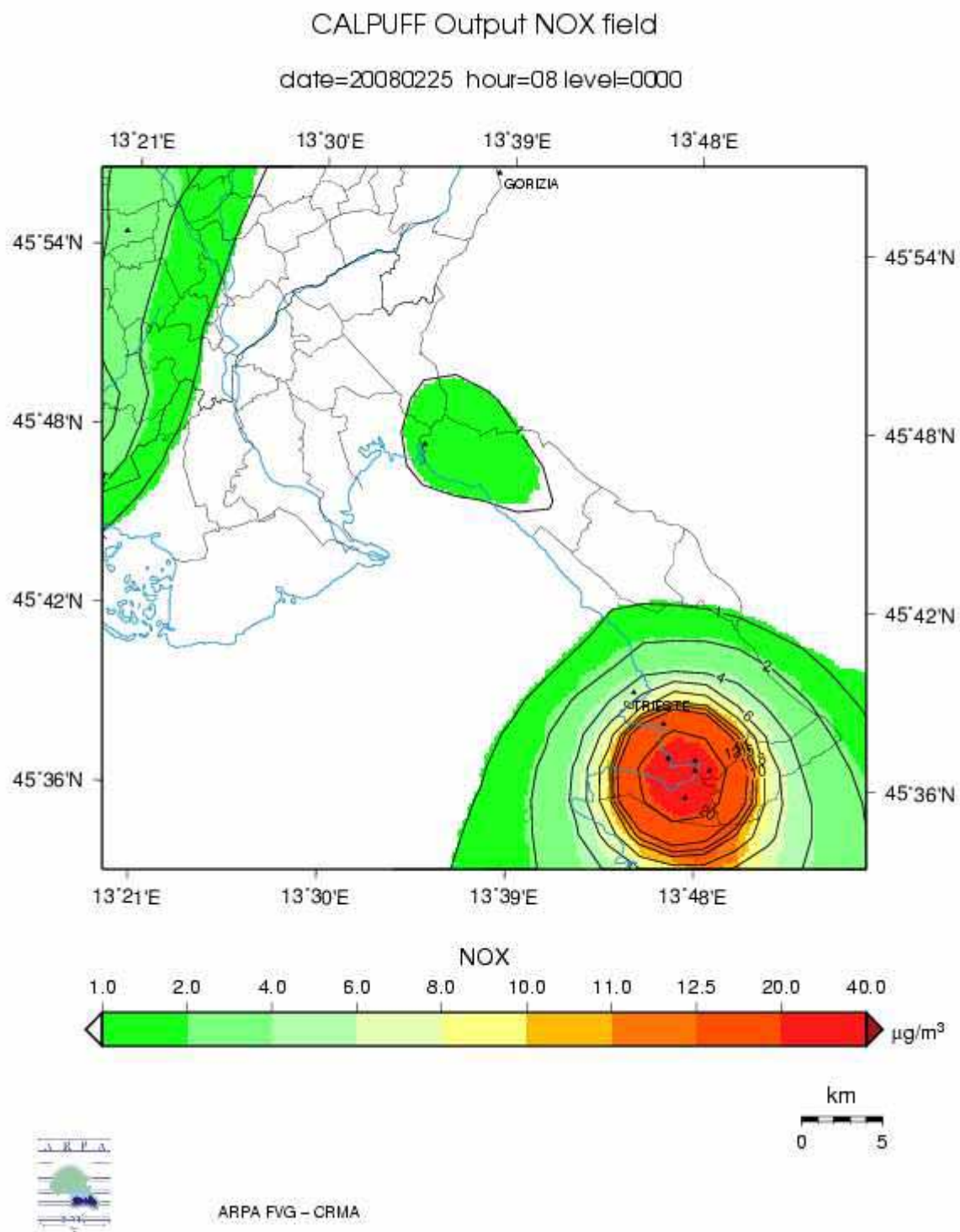
Figura 53 – Distribuzione nell'area interessata delle concentrazioni di NOx il giorno 25/02/2008 alle ore 08. Nel modello diffusionale sono state incluse tutte le sorgenti puntuali di Ossidi di Azoto.
