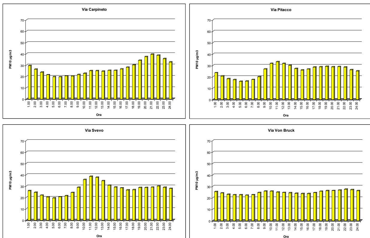
Figura 67: andamento medio orario (13/07/2007 – 11/11/2008) delle polveri sottili nelle stazioni prossime alla ferriera di Servola.
