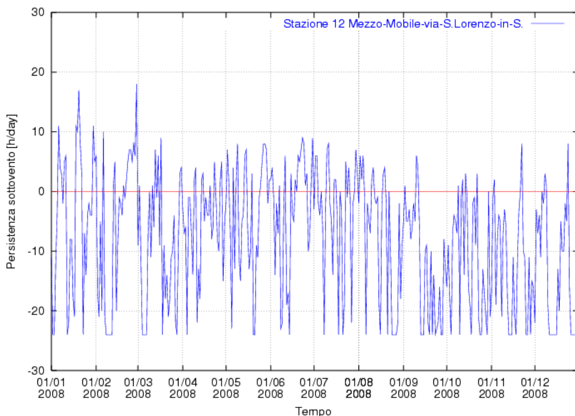
Figura 88: persistenza anemologica nella stazione di via San Lorenzo in Selva (R.F.I.).
