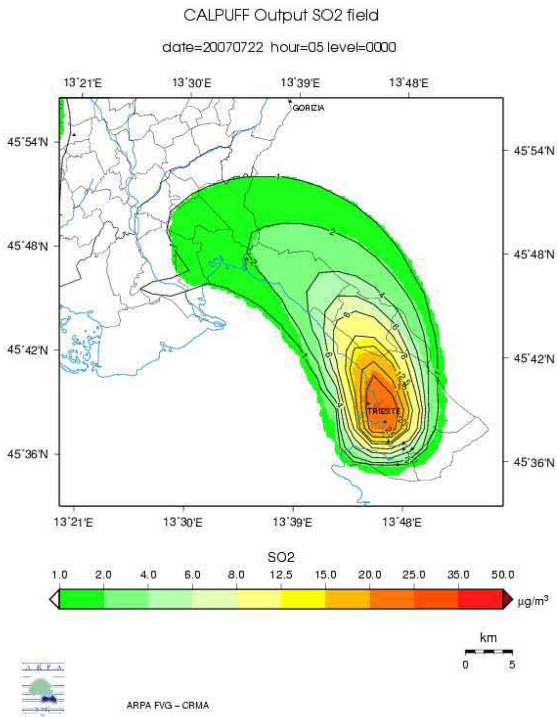
Figura 50 – Distribuzione nell'area interessata delle concentrazioni di SO 2 il giorno 22/07/2007 alle ore 05. Nel modello diffusionale sono state incluse tutte sorgenti puntuali di Ossidi di Zolfo.
