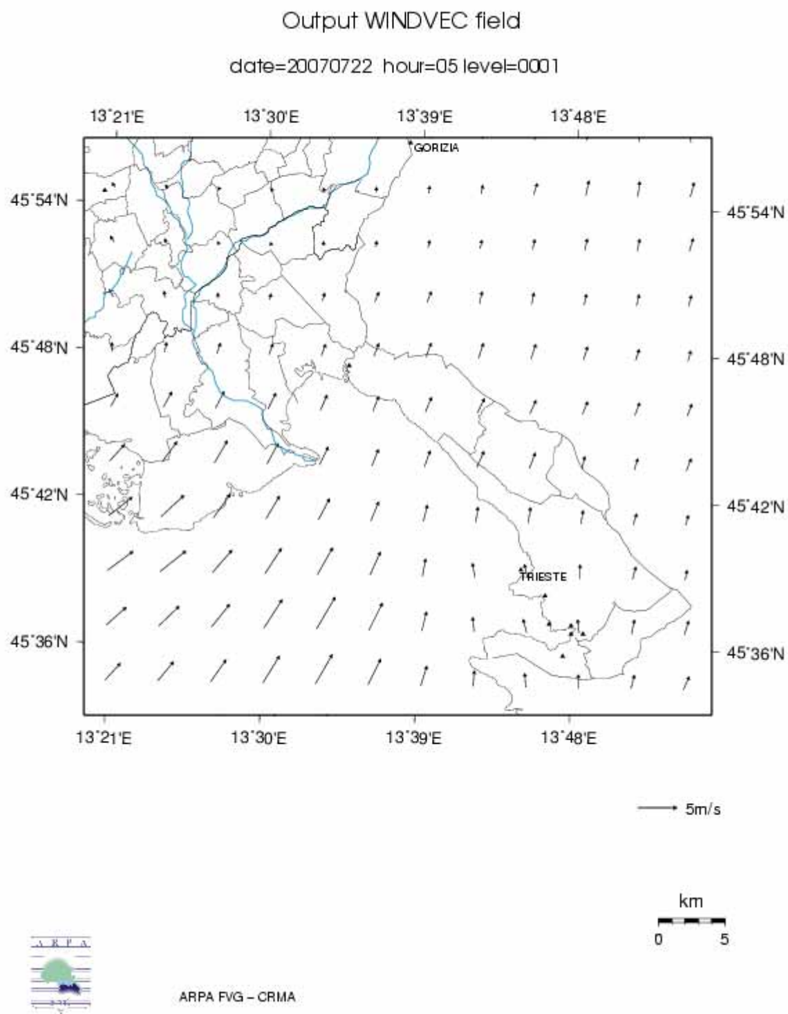
Figura 47 – Direzione ed intensità del vento rilevate il giorno 22/07/2007 alle ore 05 nell'area interessata.
