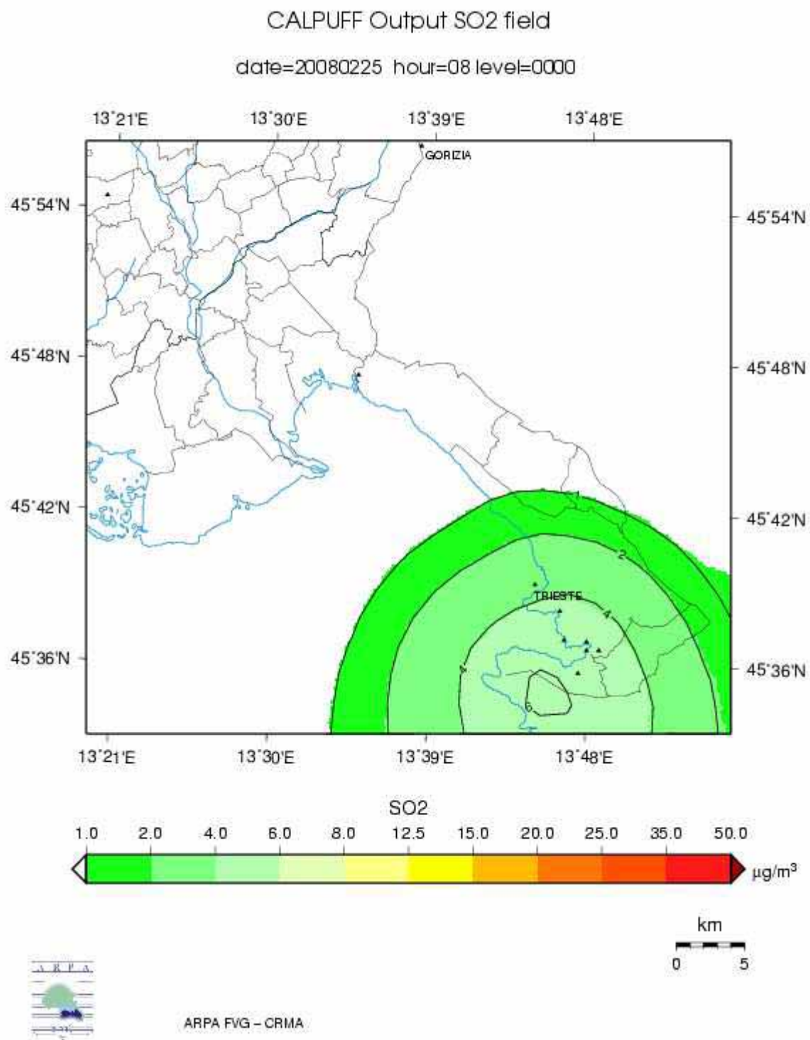
Figura 56 – Distribuzione nell'area interessata delle concentrazioni di SO 2 il giorno 25/2/2008 alle ore 08. Nel modello diffusionale sono state compute unicamente le immissioni in atmosfera di Ossidi di Zolfo provenienti dallo stabilimento di Servola.
