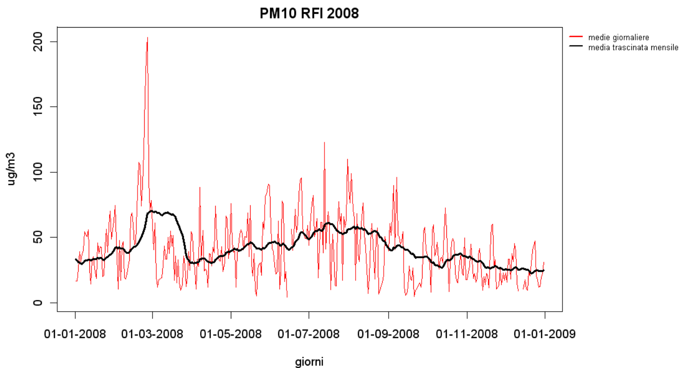
Figura 57 – Andamento delle medie traccinate mensili nell'anno 2008 nella stazione denominata R.F.I..
