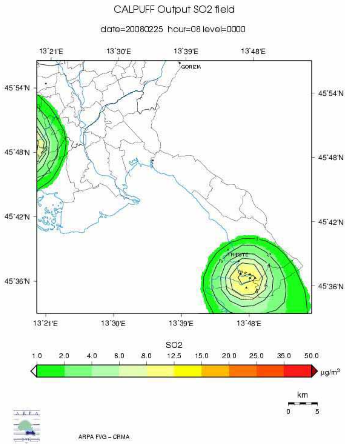
Figura 55 – Distribuzione nell'area interessata delle concentrazioni di SO 2 il giorno 25/02/2008 alle ore 08. Nel modello diffusionale sono state incluse tutte le sorgenti puntuali di Ossidi di Zolfo.
