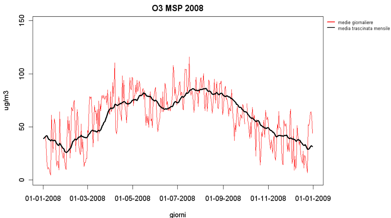
Figura 37 – Andamento delle medie traccinate mensili di Ozono nel corso dell'anno 2008 nella stazione di Monte San Pantaleone.
