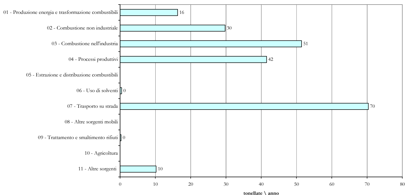
Emissione di PM 10 nel Comune di Trieste ripartite per macrosettore
