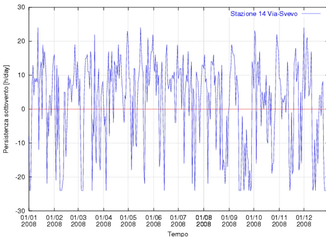
Figura 85: persistenza anemologica nella stazione di Via Svevo
