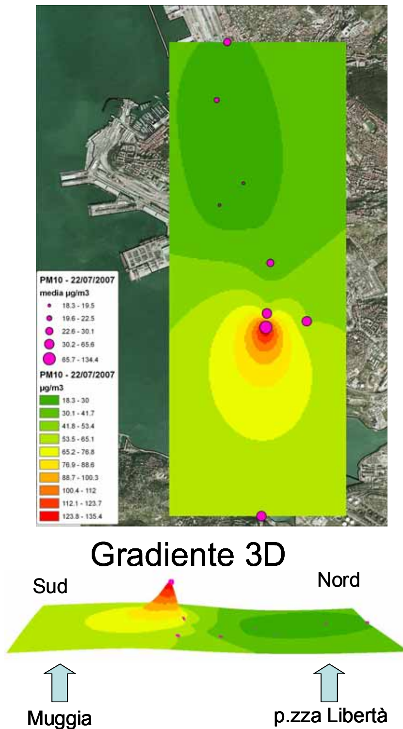
Figura 74: 22/07/2007 - interpolazione dei valori di PM10 misurati dalle centraline di ARPA.
