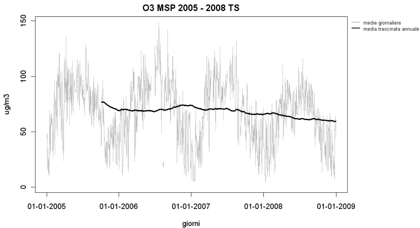
Figura 39 - Andamento dei valori delle medie trascinate annue nel periodo 2005-2008 nella stazione di Monte S. Pantaleone.
