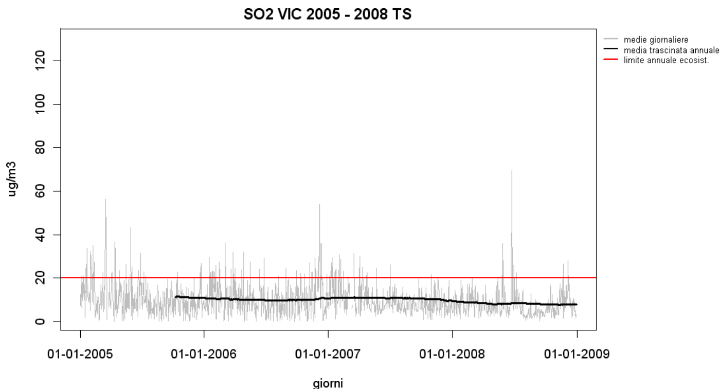
Figura 15 – Andamento delle medie trascinata annue nel periodo 2005-2008 nella stazione di piazza Vico.
