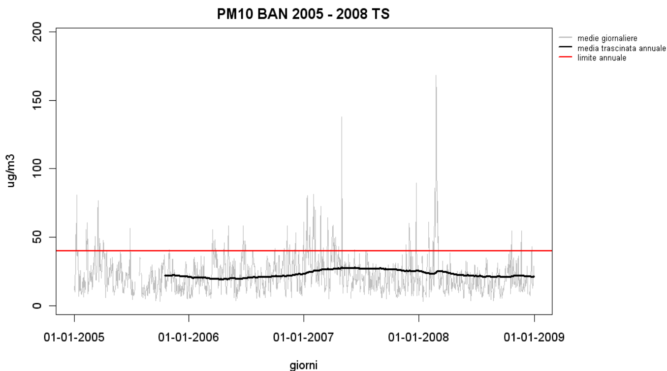
Figura 28 – Andamento delle medie trascinate annue nel periodo 2005-2008 nella stazione di via Tor Bandena.
