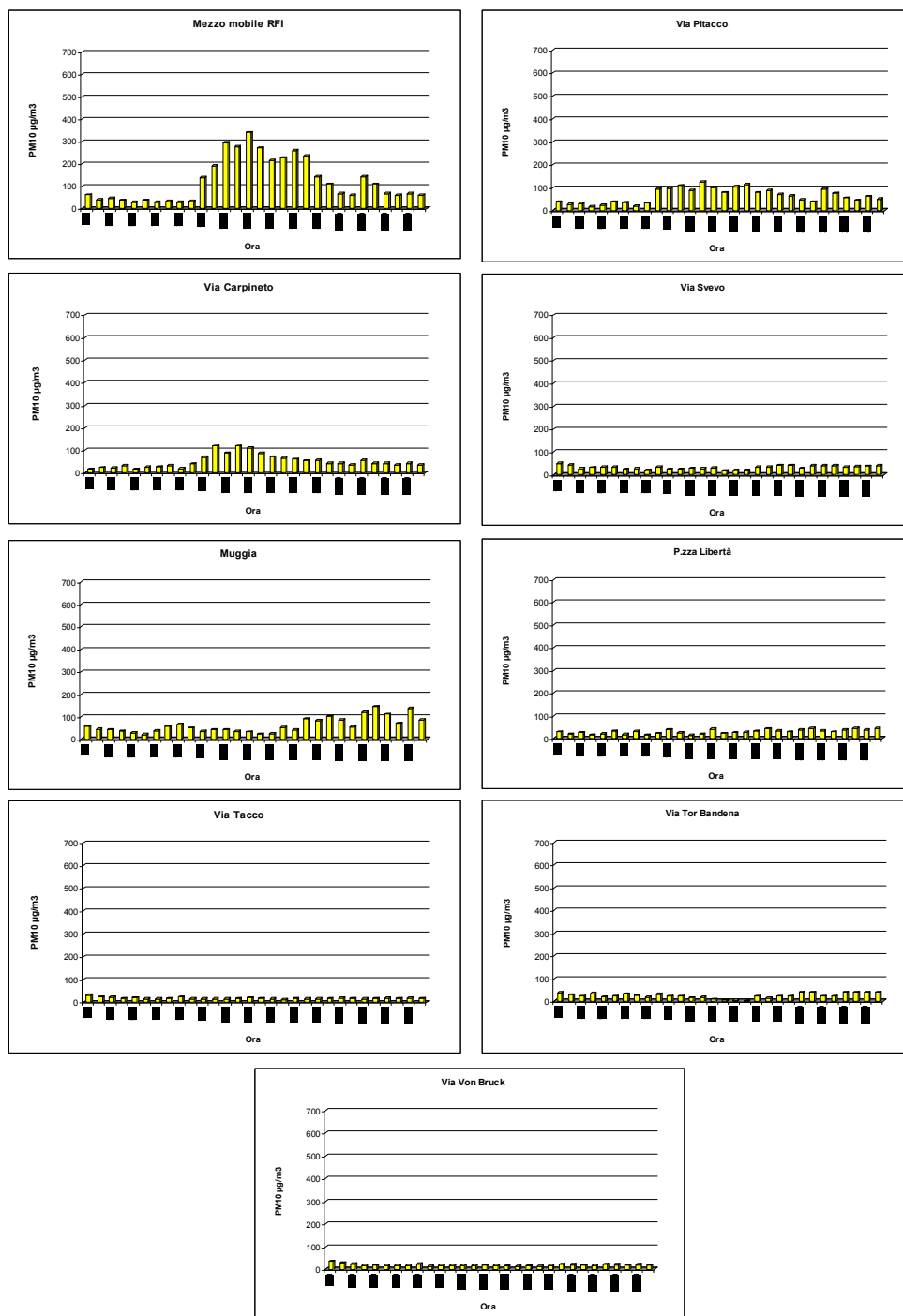
Figura 73: 22/07/2007 - andamento dei valori di PM10 nelle centraline di ARPA.
