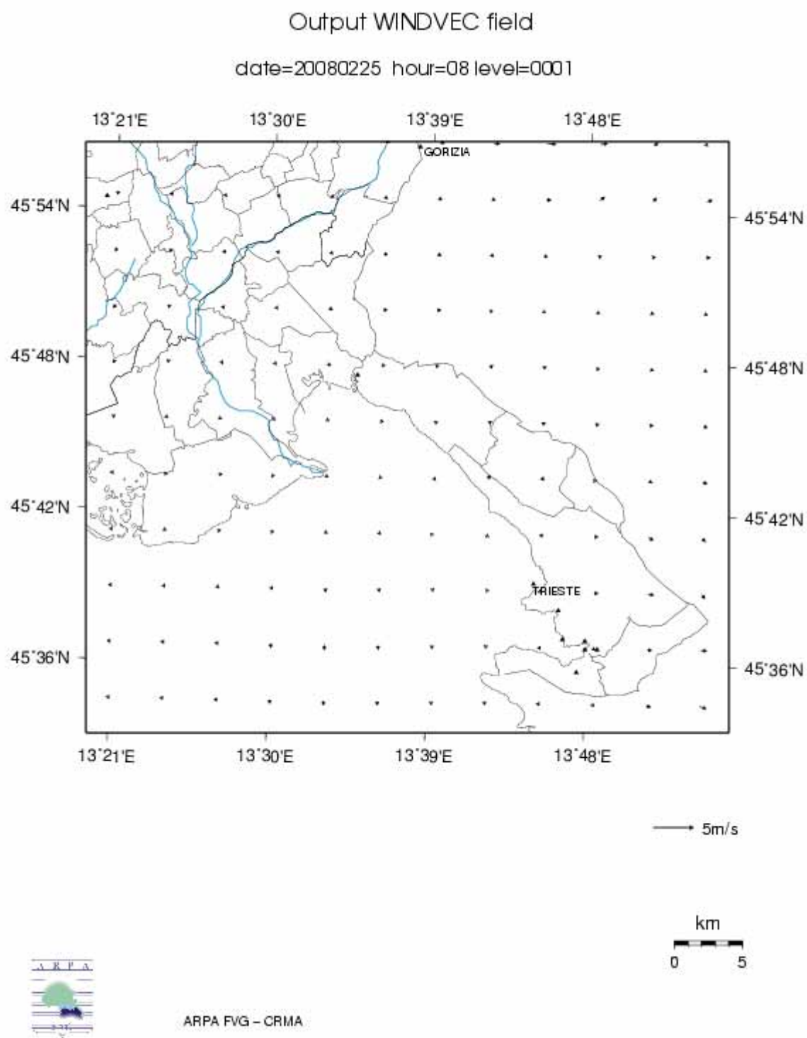
Figura 52 – Direzione ed intensità del vento rilevate il giorno 25/02/2008 alle ore 08 nell'area interessata.
