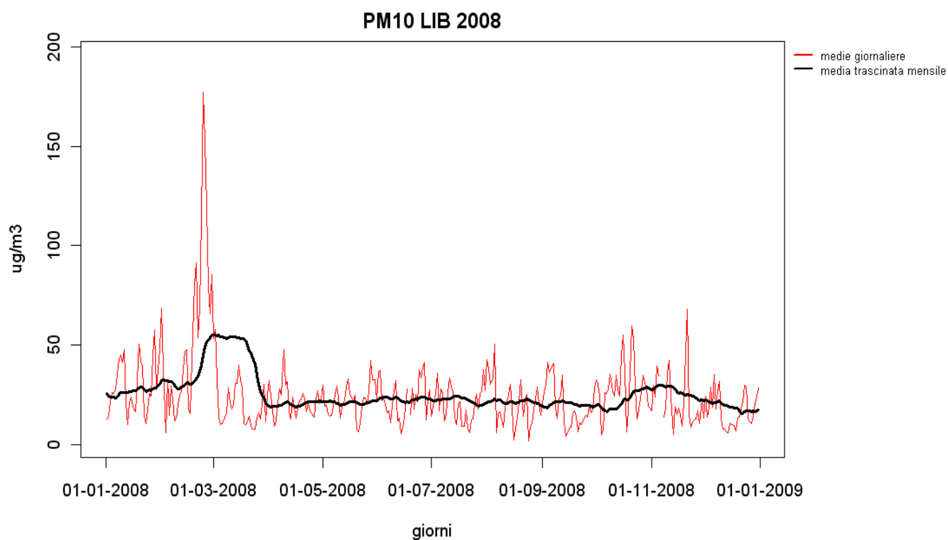
Figura 24 - Andamento delle medie trascinate mensili nell'anno 2008 nella stazione di piazza Libertà.
