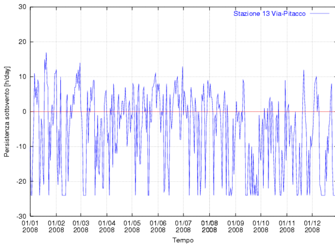
Figura 87: persistenza anomologica nella stazione di Via Pitacco
