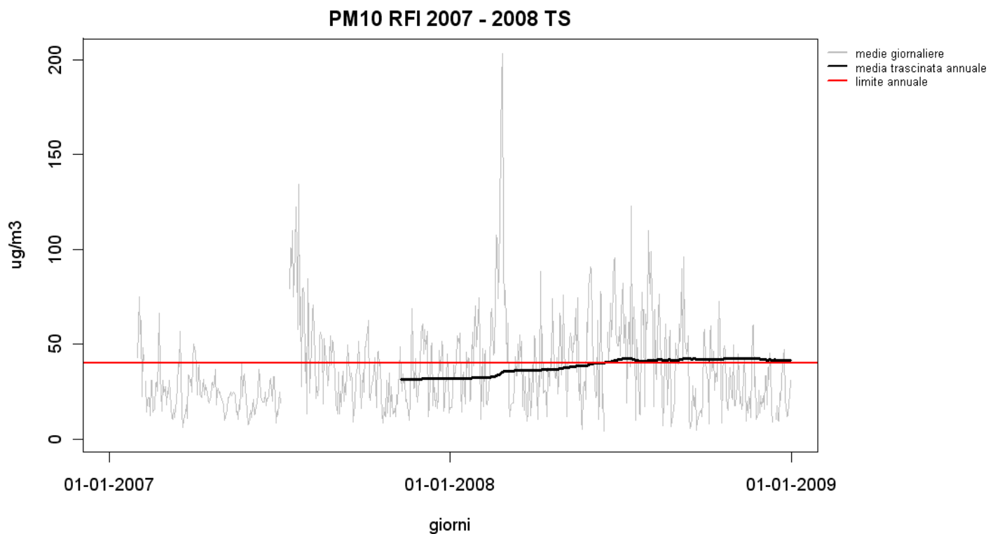
Figura 58 – Andamento delle medie traccinate annue nel periodo luglio 2007-2008 nella stazione denominata R.F.I..
