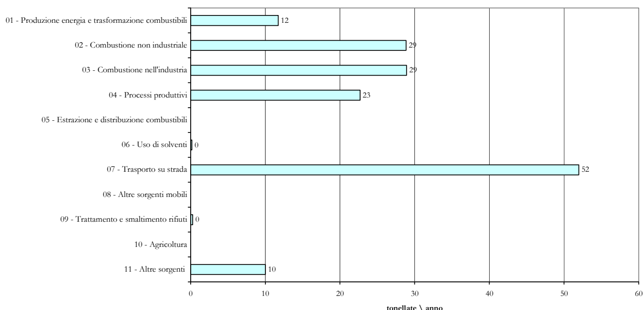
Emissione di PM 2,5 nel Comune di Trieste ripartite per macrosettore
