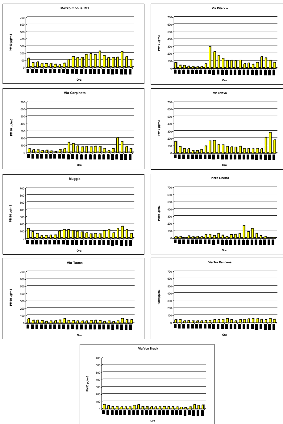
Figura 71: 19/07/2007 - andamenti orari delle concentrazioni di PM10 nelle diverse stazioni.
