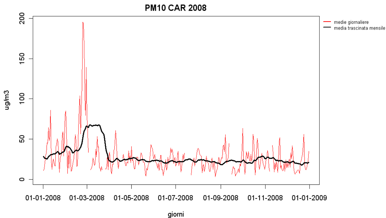
Figura 23 – Andamento delle medie trascinata mensili nell'anno 2008 nella stazione di via Carpineto.
