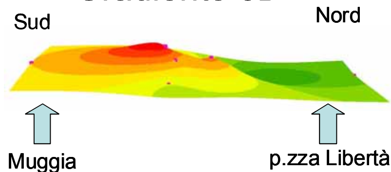
Figura 72:19/07/2007 - interpolazione dei valori di PM10 sull'area monitorata dalle centraline di ARPA.
