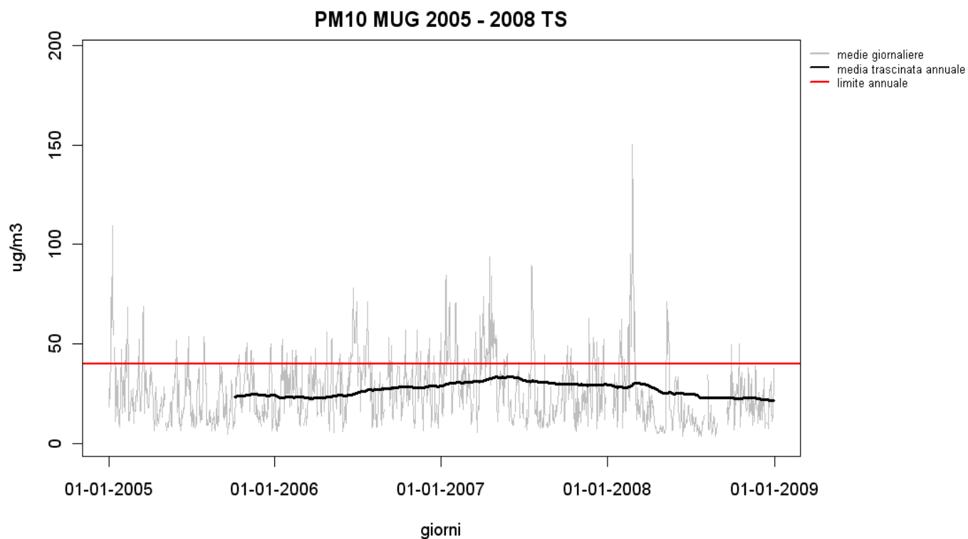
Figura 31 – Andamento delle medie trascinate annue nel periodo 2005-2008 nella stazione di Muggia.
