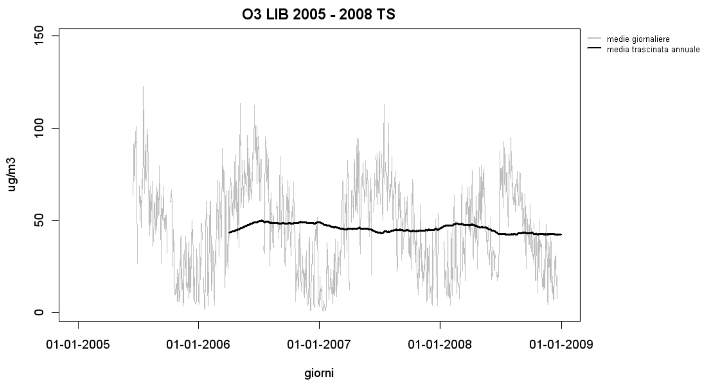
Figura 38 - Andamento dei valori delle medie trascinate annue nel periodo 2005-2008 nella stazione di piazza Libertà
