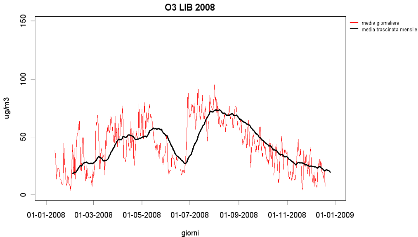
Figura 36 – Andamento delle medie traccinate mensili di Ozono nel corso dell'anno 2008 nella stazione di piazza Libertà.
