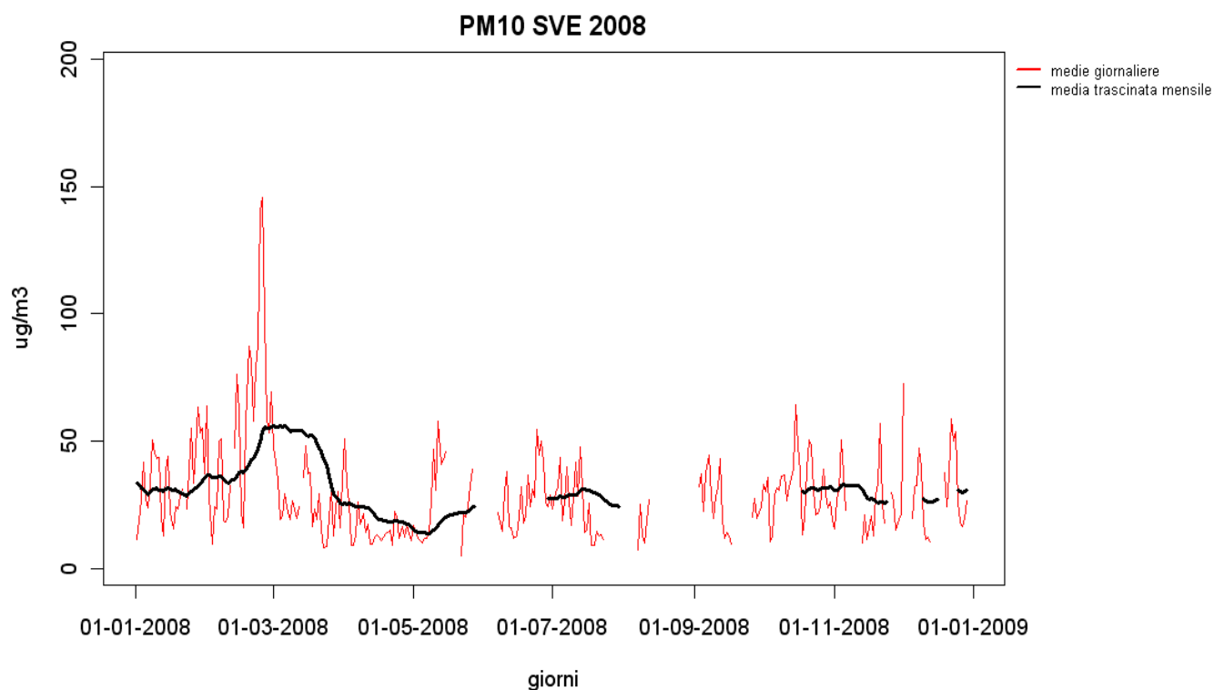
Figura 27 – Andamento delle medie trascinata mensili nell'anno 2008 nella stazione di via Svevo.
