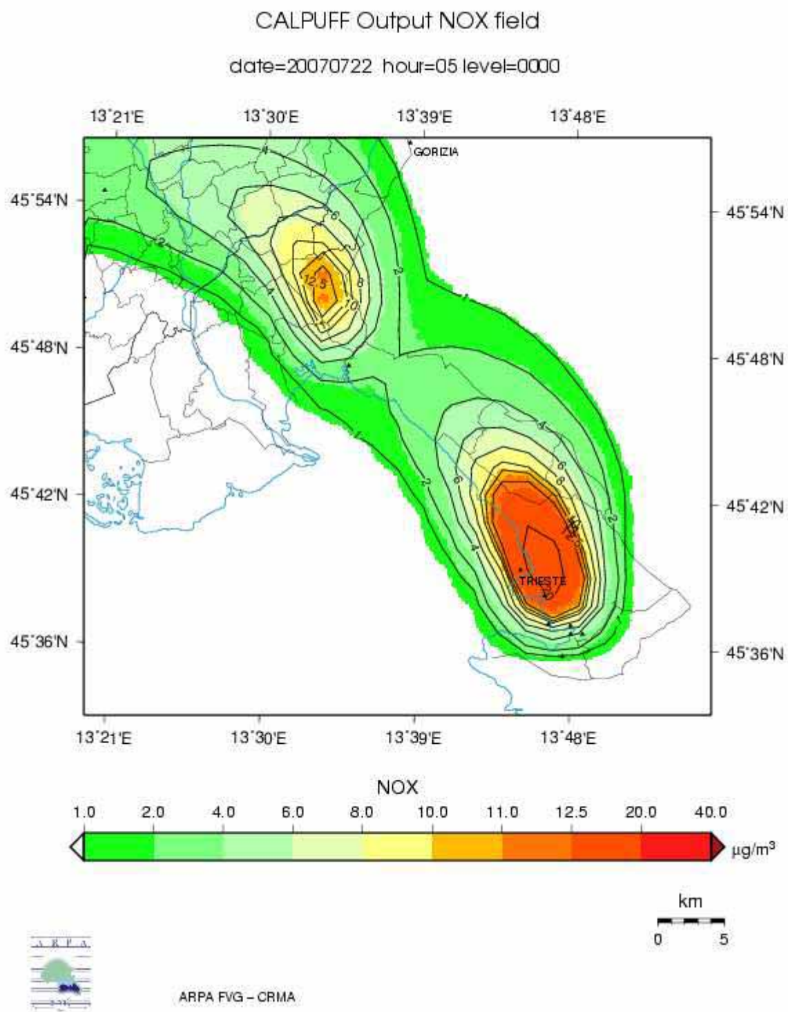
Figura 48 – Distribuzione nell'area interessata delle concentrazioni di NOx il giorno 22/07/2007 alle ore 05. Nel modello diffusionale sono state incluse tutte le sorgenti puntuali di Ossidi di Azoto.
