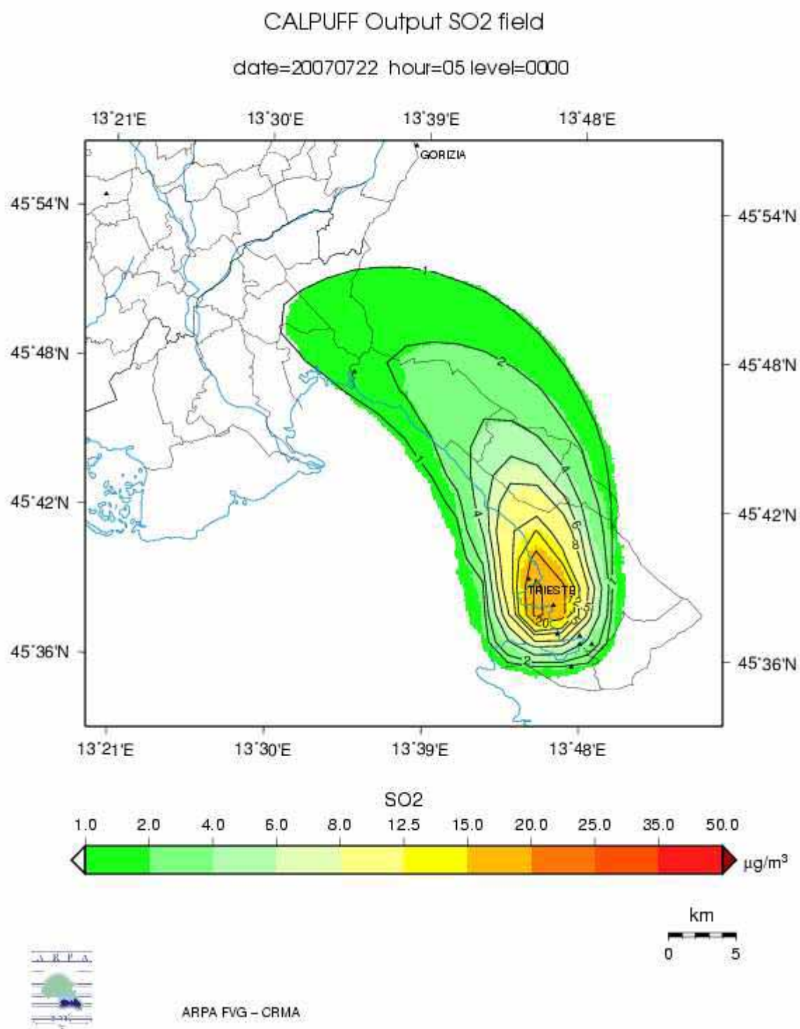
Figura 51 – Distribuzione nell'area interessata delle concentrazioni di SO 2 il giorno 22/07/2007 alle ore 05. Nel modello diffusionale sono state compute unicamente le immissioni in atmosfera di Ossidi di Zolfo provenienti dallo stabilimento di Servola.
