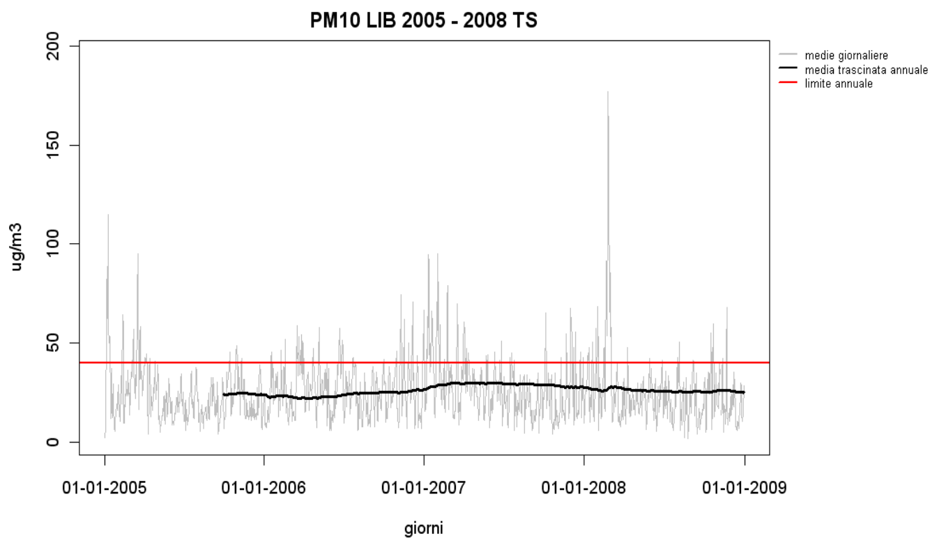
Figura 30 - Andamento delle medie trascinate annue nel periodo 2005-2008 nella stazione di piazza Libertà.
