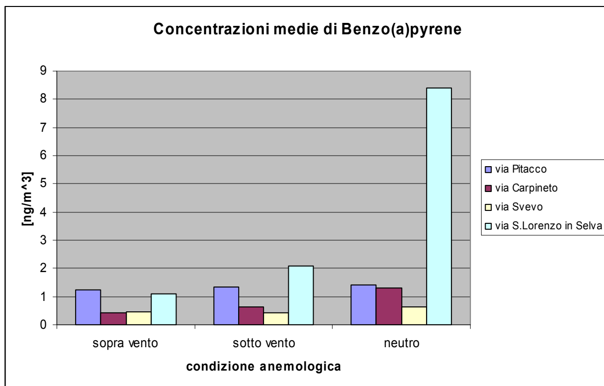
Figura 89: medie delle concentrazioni di BaP per le stazioni di via Pitacco, via Carpineto, via Svevo e via S. Lorenzo in Selva (mezzo mobile R.F.I.) nelle diverse condizioni anemologiche
