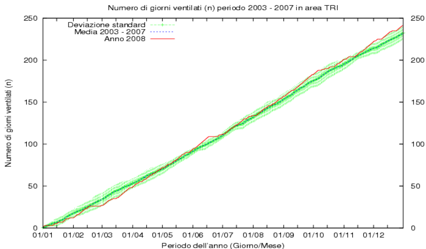
Figura 2– Cumulata media di giorni ventosi (velocità media maggiore a 2 m/s) nel periodo 2003-2007(linea blu) e nell'anno 2008 Linea rossa). L'ombreggiatura verde indica l'intervallo corrispondente a una deviazione standard.
