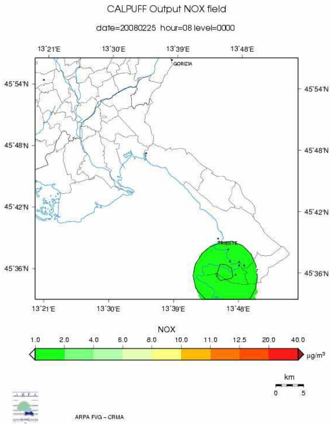
Figura 54 – Distribuzione nell'area interessata delle concentrazioni di NOx il giorno 25/02/2008 alle ore 08. Nel modello diffusionale sono state compute unicamente le immissioni in atmosfera di Ossidi di Azoto provenienti dallo stabilimento di Servola.
