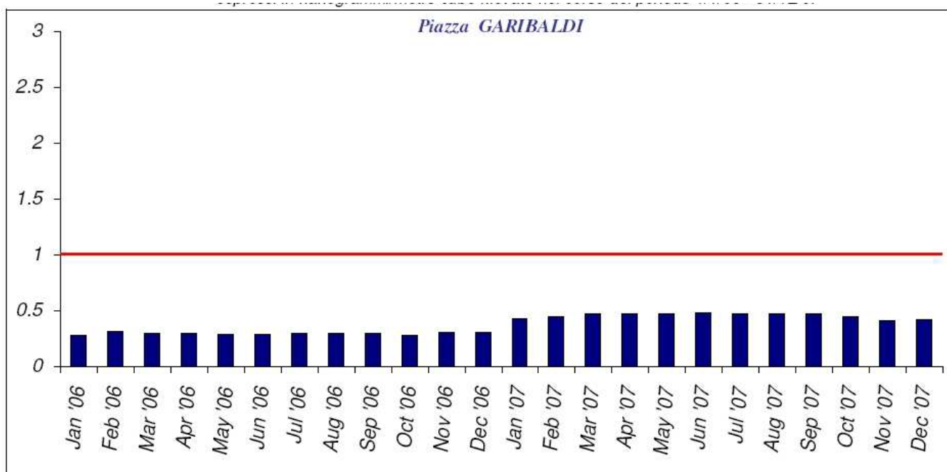
Figura 44 - Andamento delle concentrazioni di Benz(a)pyrene, espresse come media mobile, rilevate in piazza Garibaldi nel periodo 1/1/2006 – 31/12/2007.
