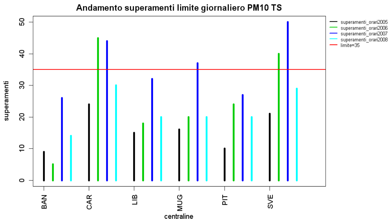
Figura 35 – Andamento del numero di superamenti del valore limite giornaliero nel periodo 2005-2008.
