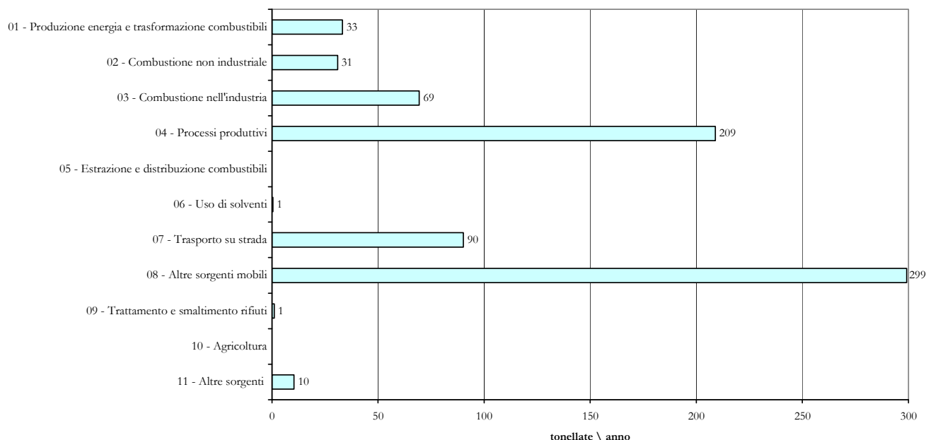
Emissione di PTS nel Comune di Trieste ripartite per macrosettore
