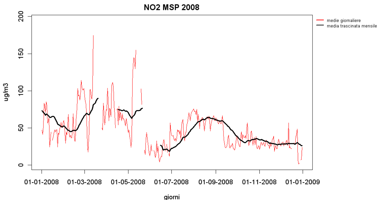
Figura 18 – Andamento delle medie trascinata mensili nel 2008 nella stazione di Monte San Pantaleone.
