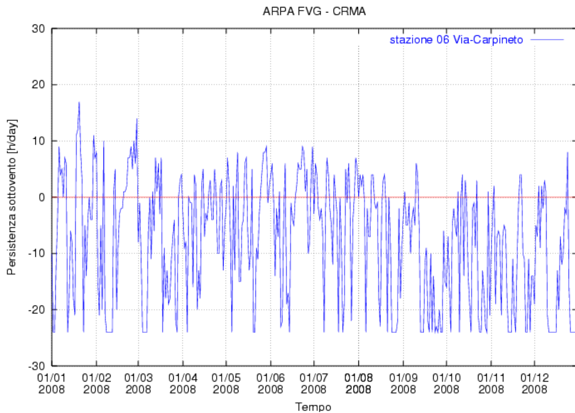
Figura 86: persistenza anomologica nella stazione di Via Carpineto
