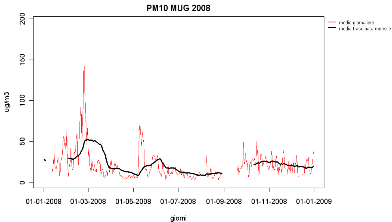
Figura 25- Andamento delle medie trascinate mensili nell'anno 2008 nella stazione di Muggia.
