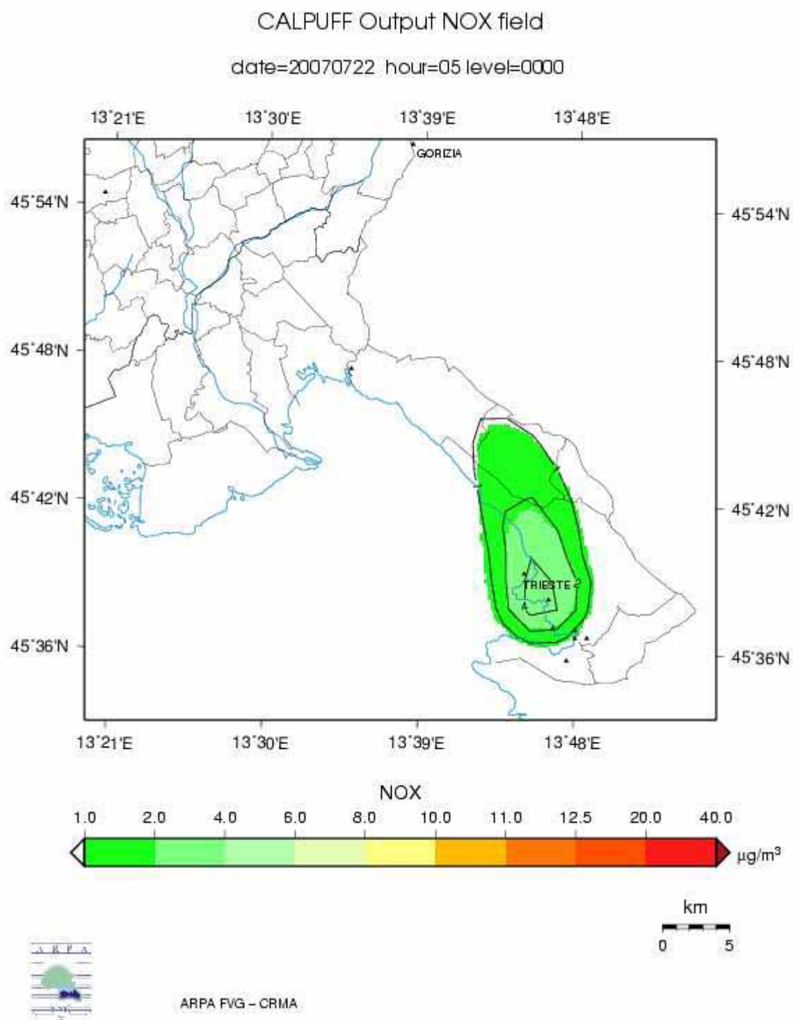
Figura 49 – Distribuzione nell’area interessata delle concentrazioni di NOx il giorno 22/07/2007 alle ore 05. Nel modello diffusionale sono state computeate unicamente le immissioni in atmosfera di Ossidi di Azoto provenienti dallo stabilimento di Servola.
