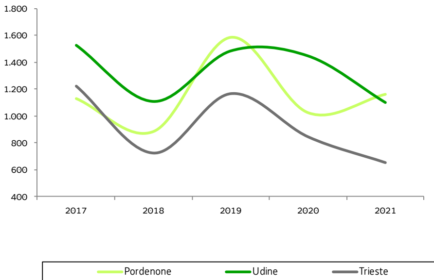
Graf. 2.2 - FVG PRECIPITAZIONI TOTALI ANNUE COMUNI CAPOLUOGO (millimetri) - Anni 2017-2021
