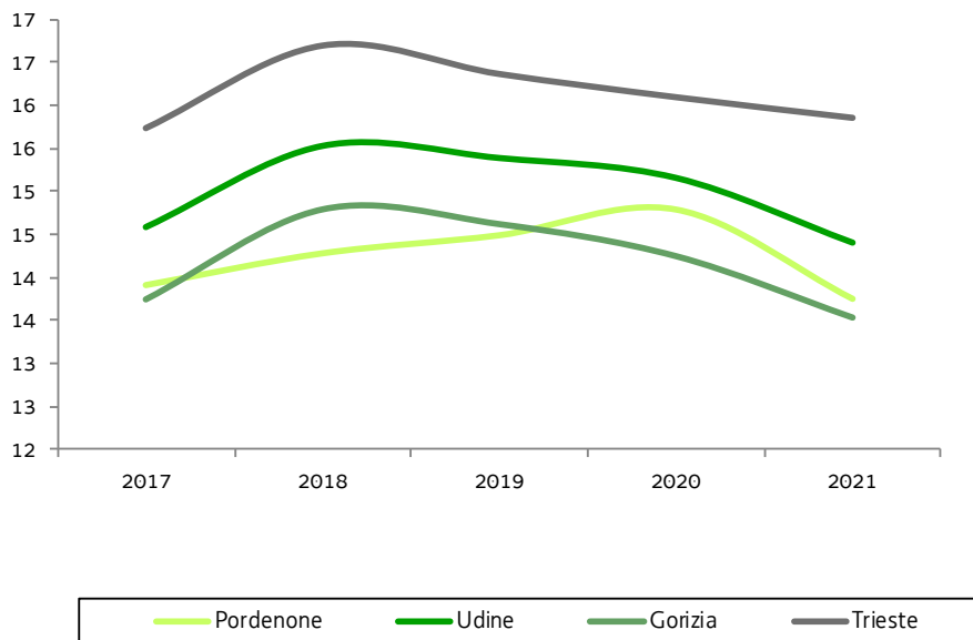
Graf. 2.1 - FVG TEMPERATURA MEDIA ANNUA COMUNI CAPOLUOGO (gradi Celsius) - Anni 2017-2021
