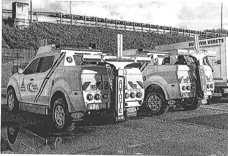
Pick up attrezzati con forche per il sollevamento dei veicoli
