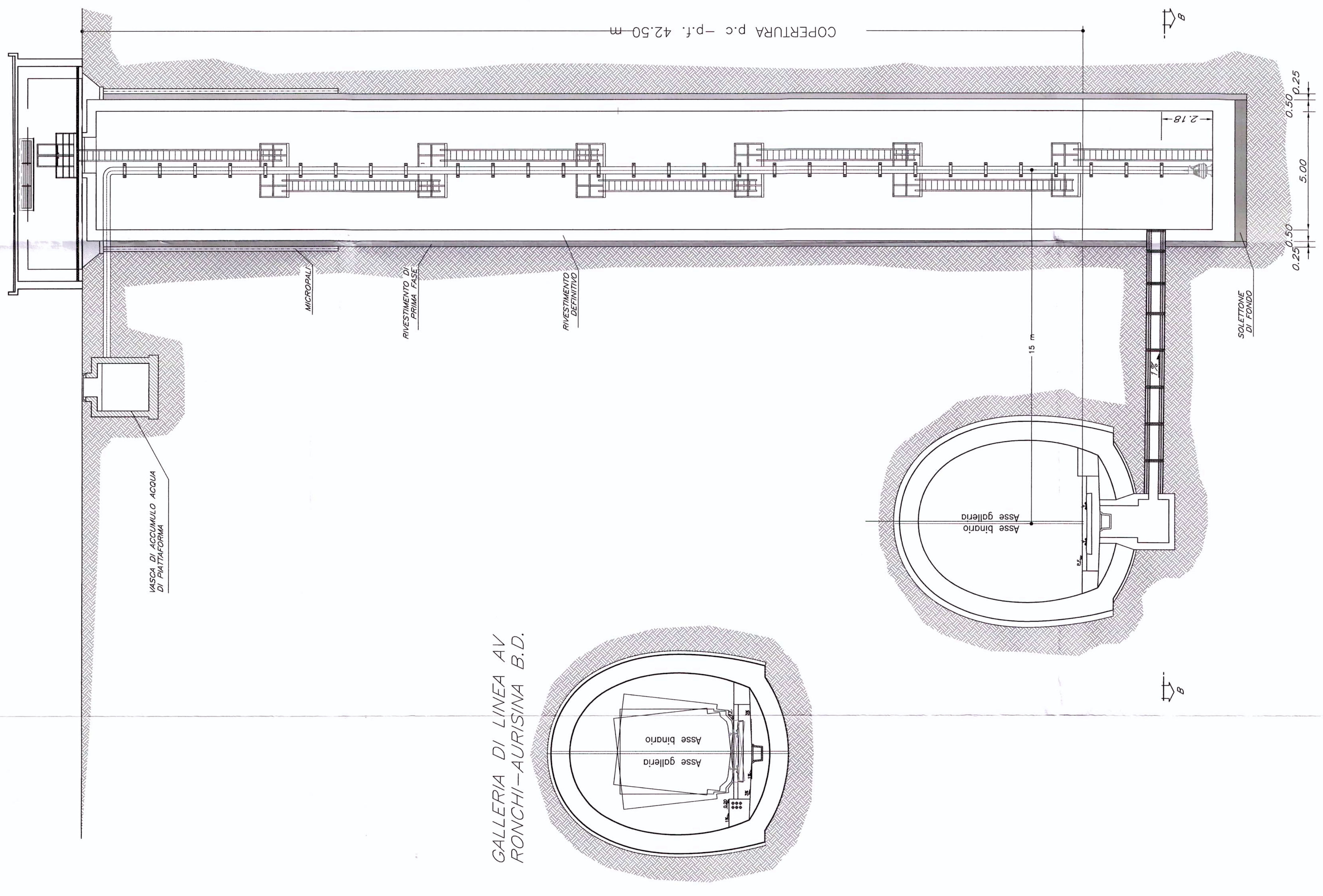
SEZIONE A-A SCALA 1/100 INTERCONNESSIONE AURISINA B.D.
