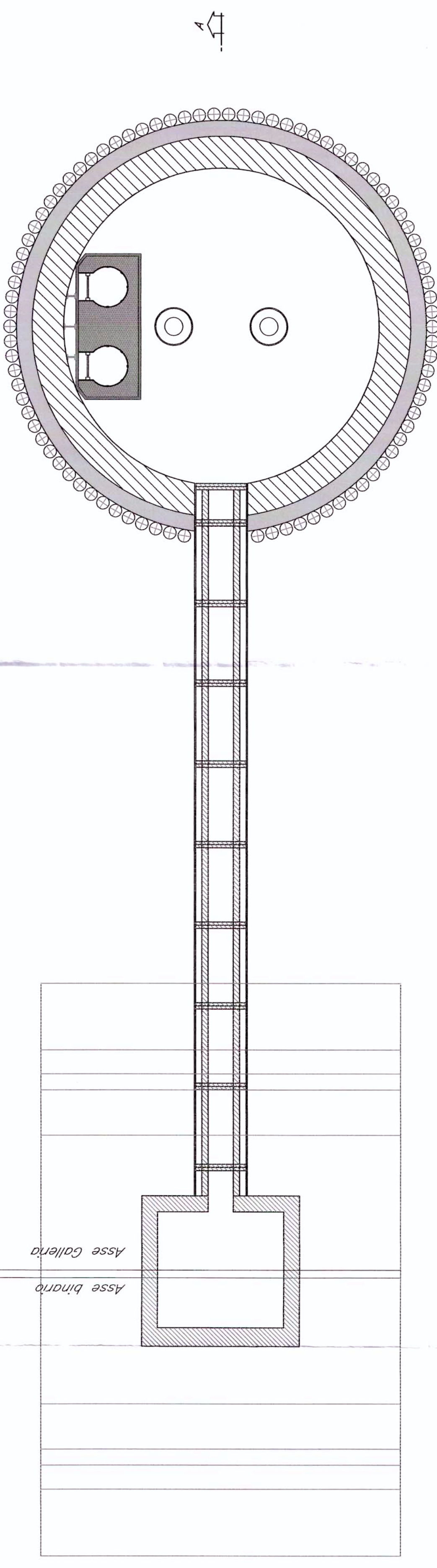
SEZIONE B-B SCALA 1:50
