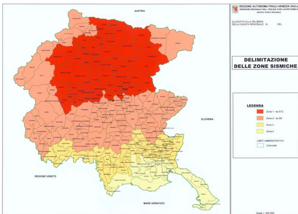
Figura 1.2. Delimitazione delle zone sismiche
